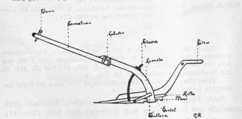
Abb. 177. Andere Pflugform aus dem katalanischen Gebiet.
