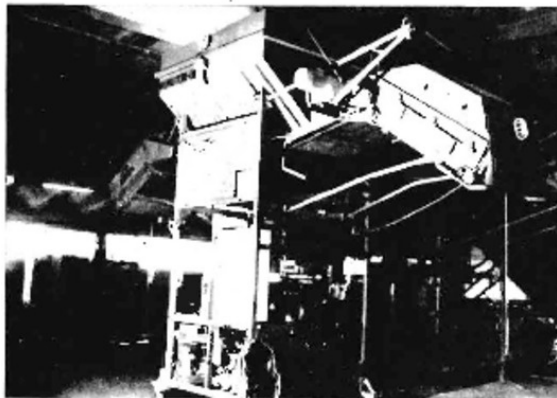
Pflanzkartoffelbeizer „Gumotex-60“
